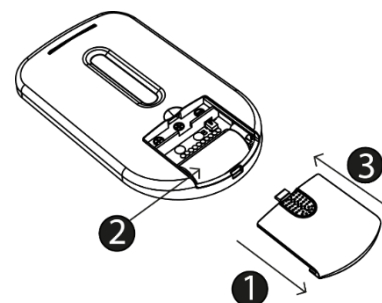
Abbildung 2: Einfügen der Batterie
